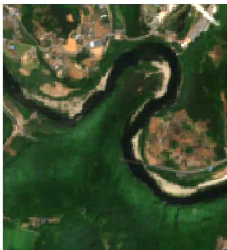
Sentinel-2 위성영상 (강원도 영월군 청령포)
